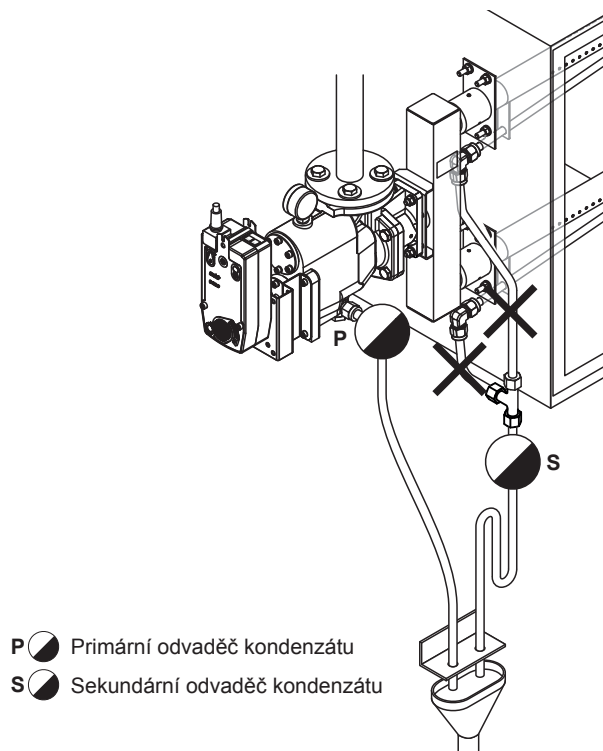
Obr. 50: Nesprávně provedený odvod kondenzátu
