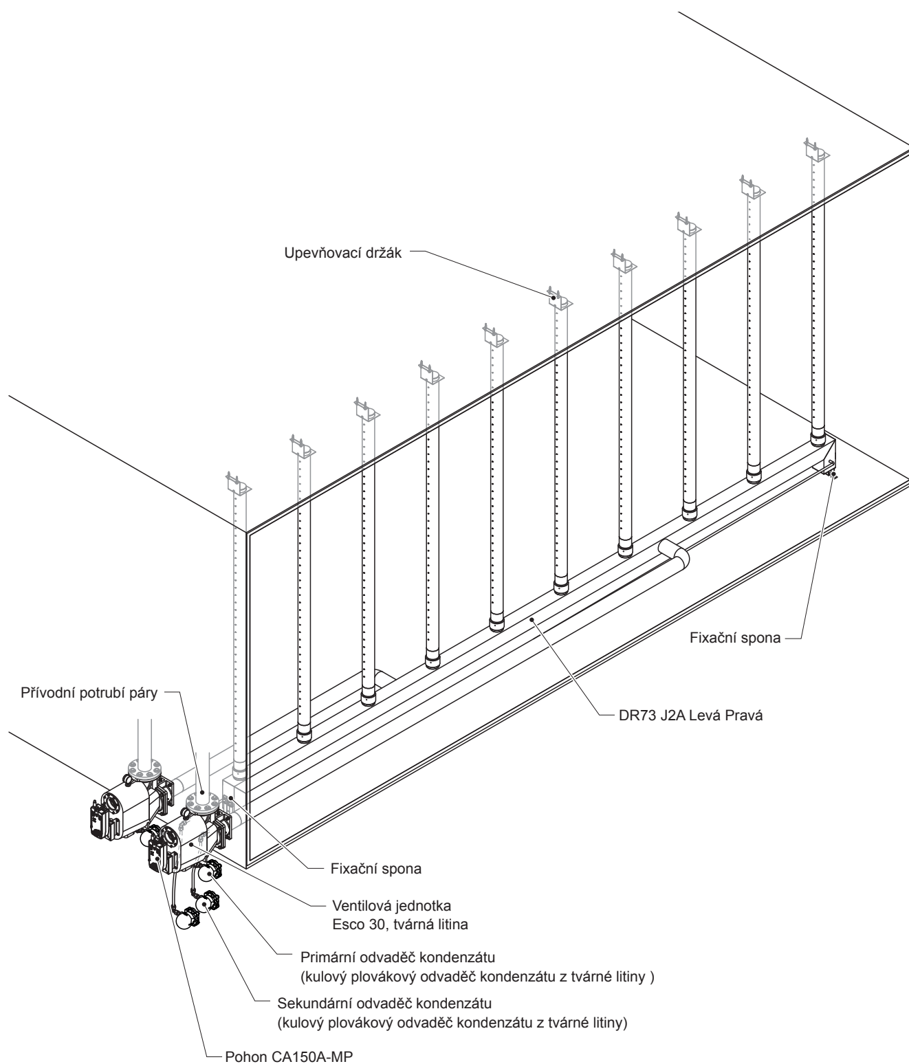
Obr. 6: Přehled instalace Condair Esco 30 tvárná litina s DR73 J2A Levá Pravá
