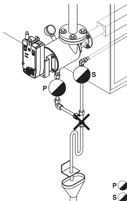
Obr. 48: Nesprávně provedený odvod kondenzátu
