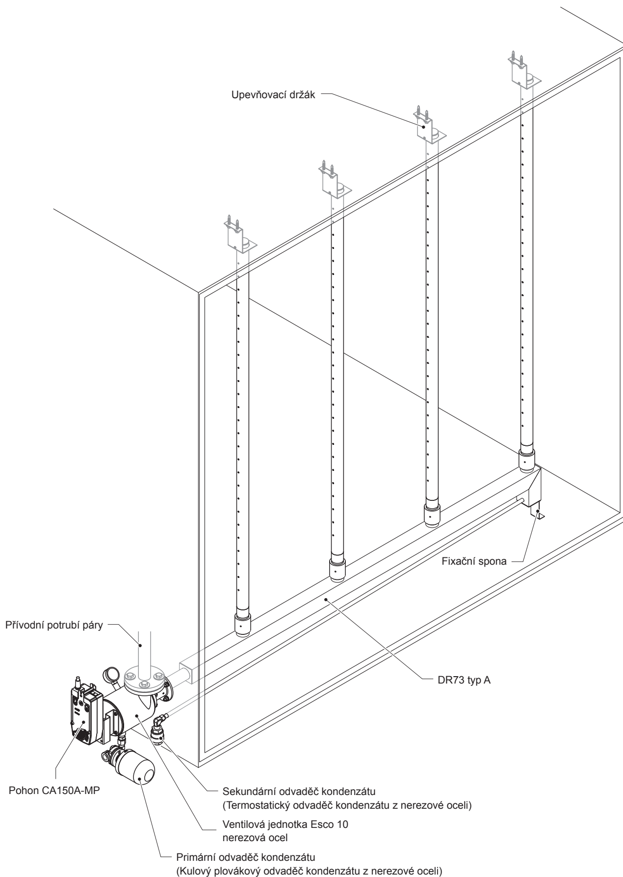
Obr. 4: Přehled instalace Condair Esco 10 nerezová ocel s DR73 typ A
