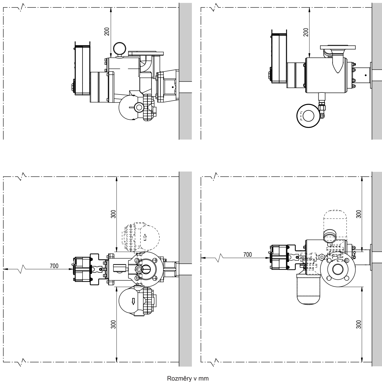
Obr. 57: Kolem ventilové jednotky je třeba udržovat mezery
