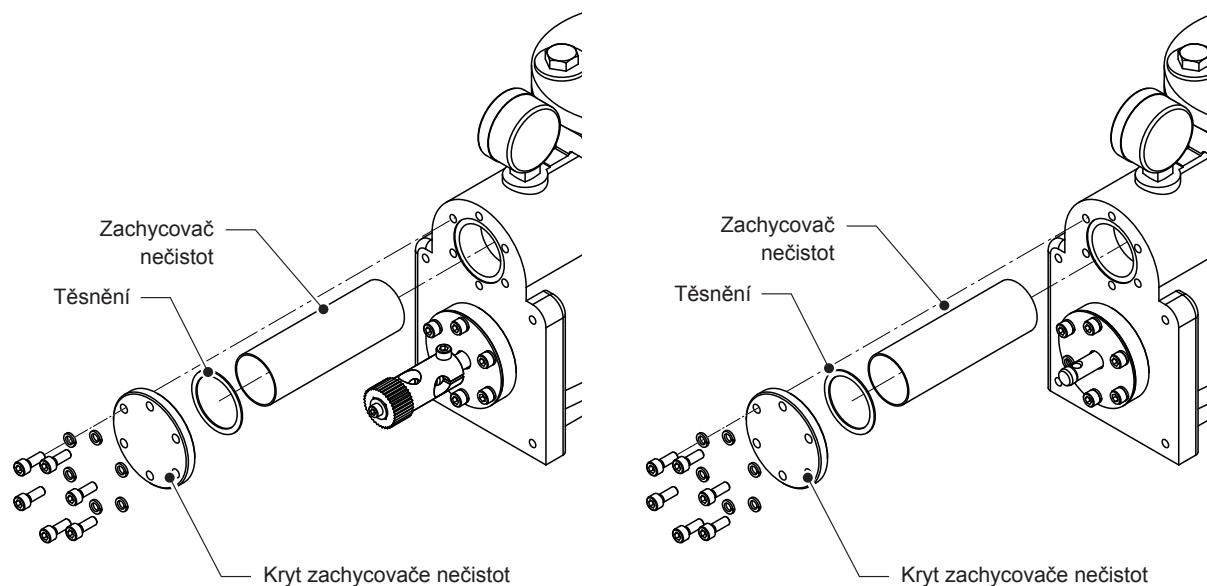
Obr. 56: Demontáž zachycovače nečistot
