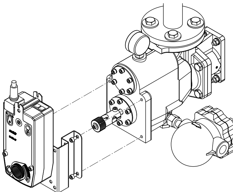
Obr. 54: Demontáž elektrického pohonu
