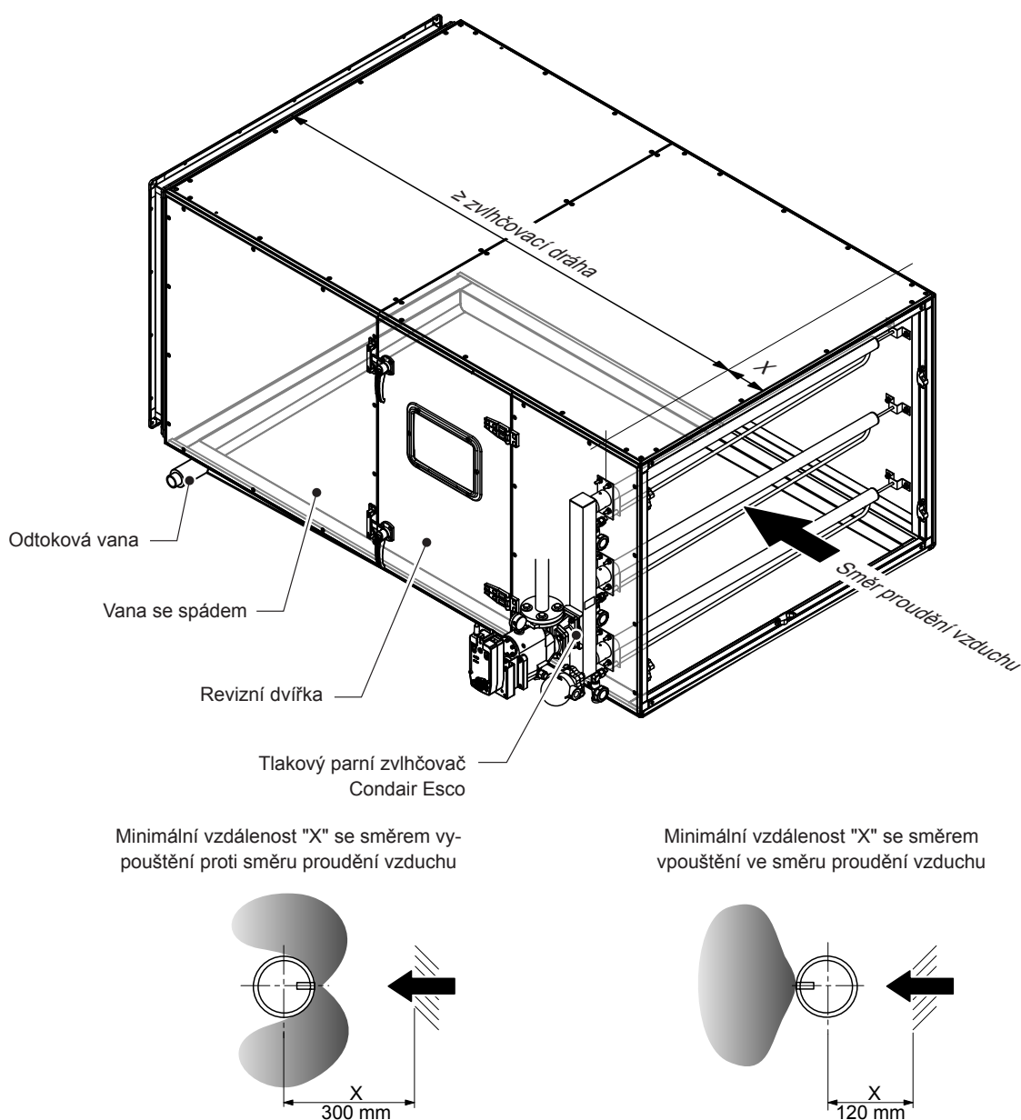
Obr. 27: Vzduchovod/VZT jednotka s DL40: Vzdálenost od předřazených a navazujících překážek
