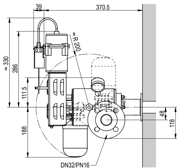
Obr. 66: Rozměrový výkres Esco 10 nerezová ocel s kulovým plovákovým odváděčem kondenzátu s pneumatickým pohonem Sauter AK41
