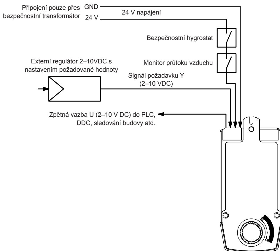
Obr. 34: Schéma pohonu CA150A-MP
