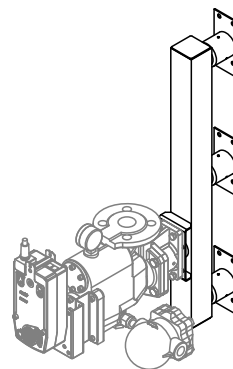
POHLED Z BOKU
