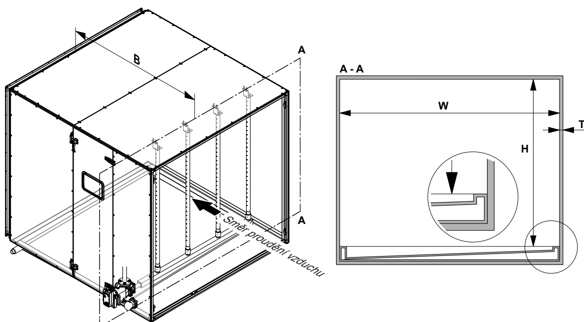
Obr. 51: Rozměry vzduchovodu/VZT jednotky
