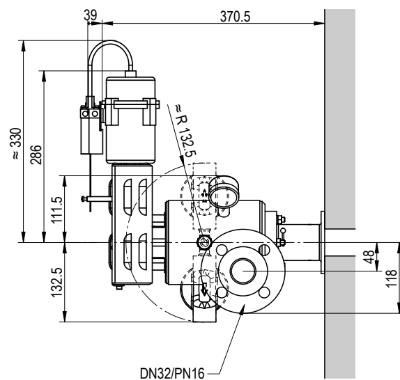
Obr. 67: Rozměrový výkres Esco 10 nerezová ocel se zvonovým plovákovým odváděčem kondenzátu s pneumatickým pohonem Sauter AK41
