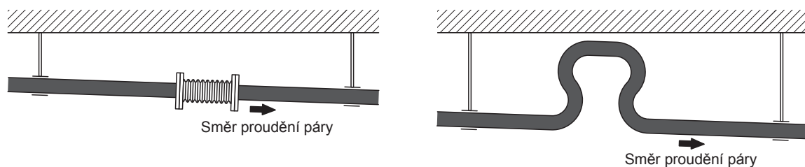
Obr. 43: Závěsy / kompenzátory
