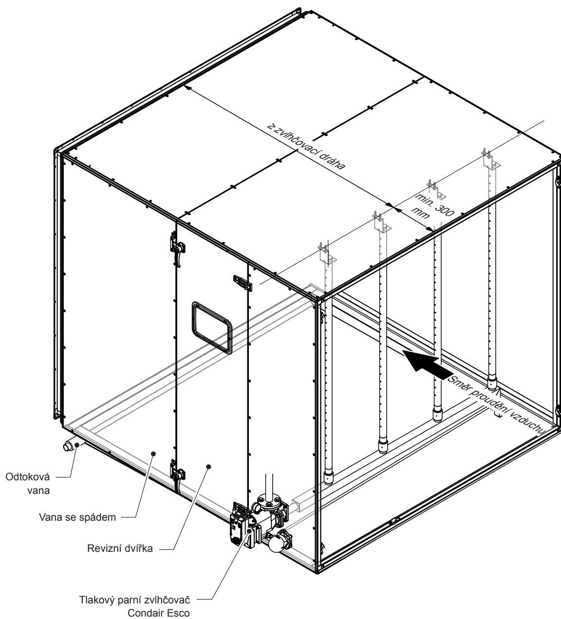
Obr. 28: Vzduchovod/VZT jednotka s DR73: Vzdálenost od předřazených a navazujících překážek
