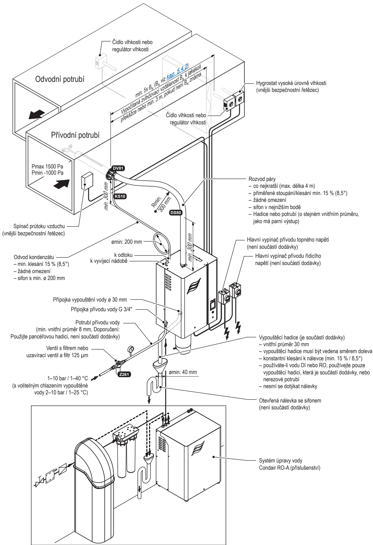
Obr. 7: Typická instalace potrubního zvlhčování
