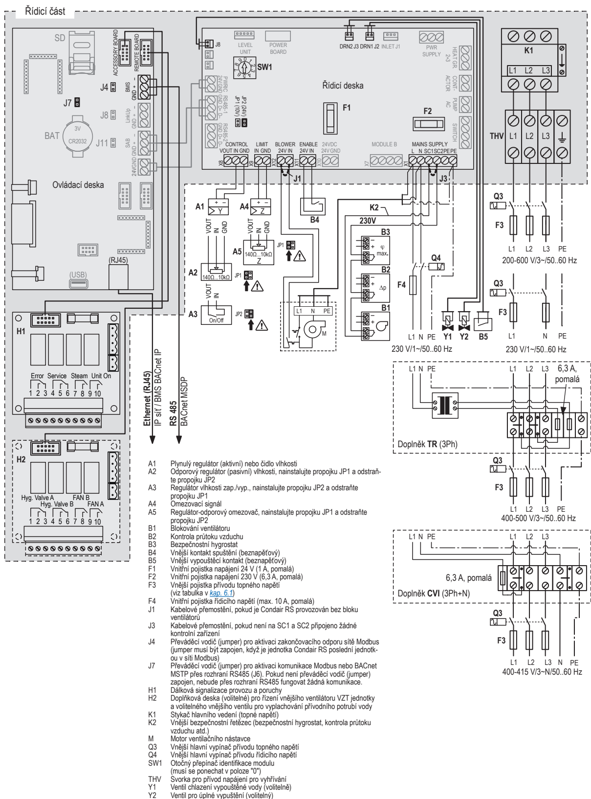
Obr. 25: Schéma elektrického zapojení samostatných malých ("S") a středních ("M") jednotek Condair RS (5–40 kg/h)
