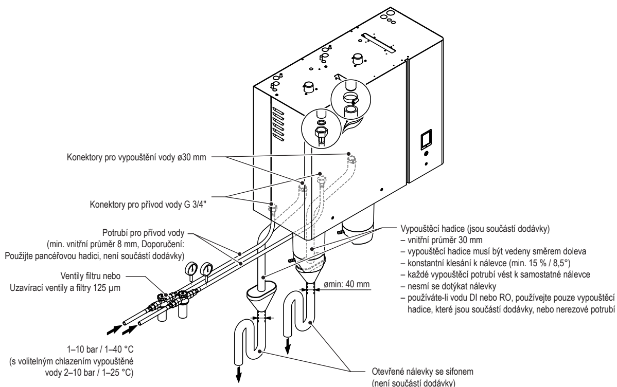
Obr. 20: Přehled vodoinstalace u samostatné velké jednotky
