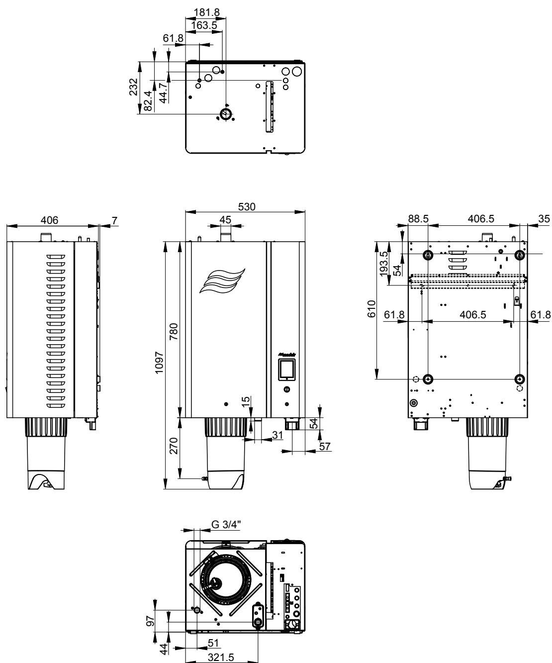
Obr. 30: Výkres rozměrů "střední" jednotky (rozměry v mm)
