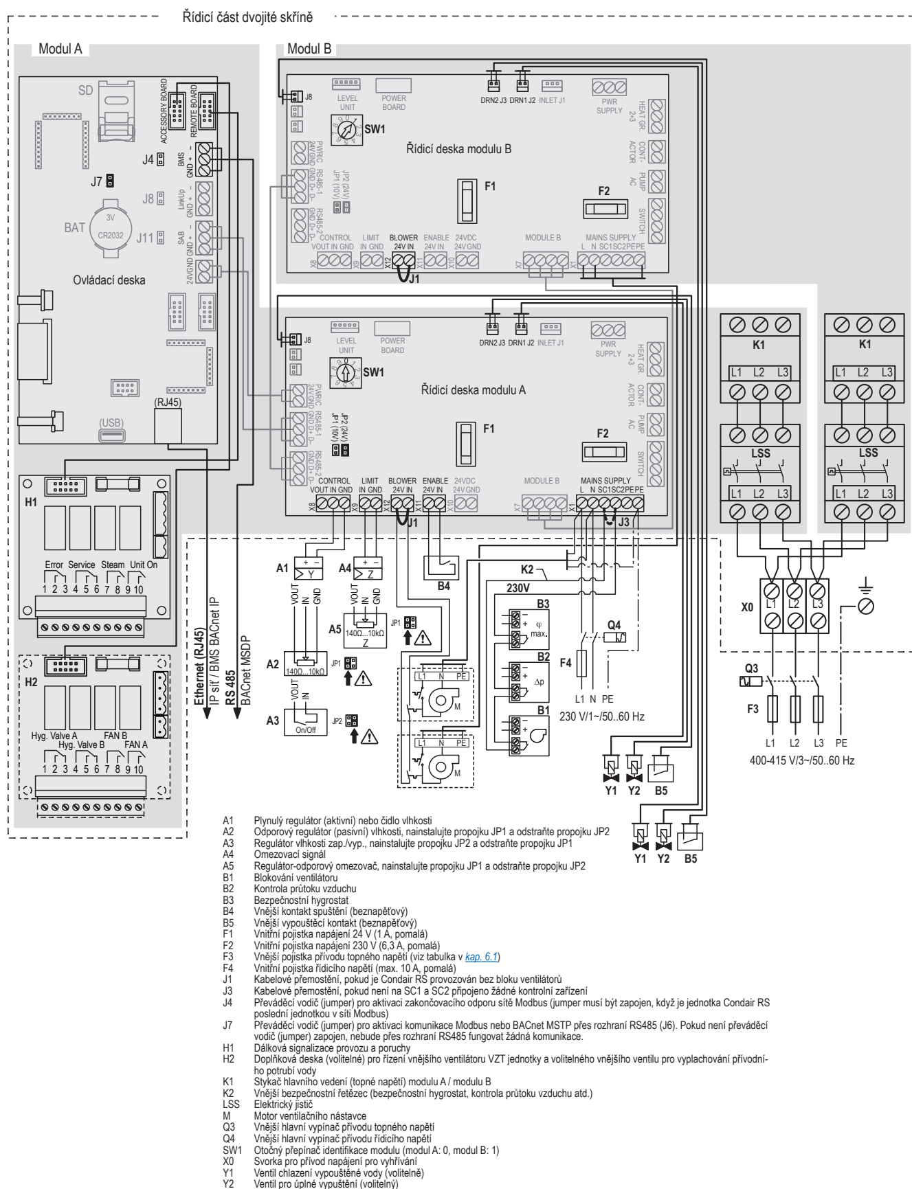
Obr. 26: Schéma elektrického zapojení samostatných velkých ("L") jednotek Condair RS 50–80 kg/h
