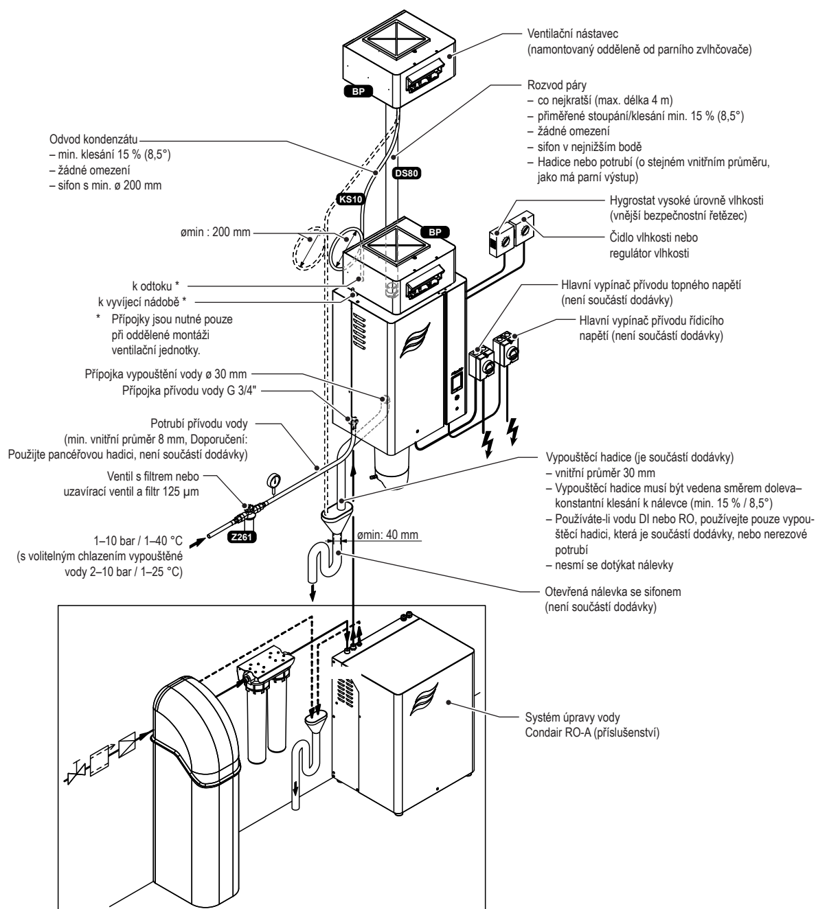
Obr. 8: Typická instalace prostorového zvlhčování
