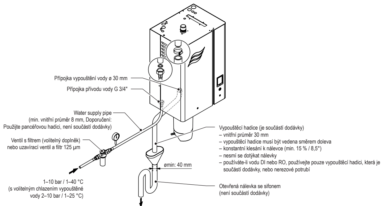
Obr. 19: Přehled vodoinstalace u samostatné malé a střední jednotky
