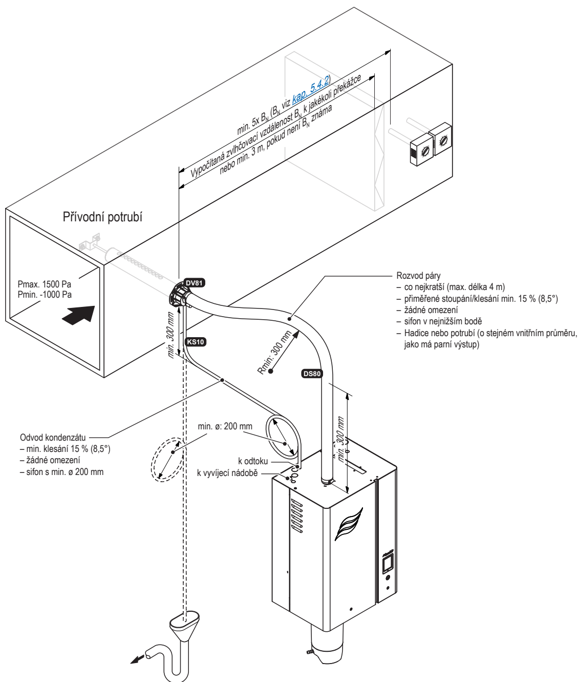
Obr. 12: Přehled instalace parního systému u potrubního zvlhčování
