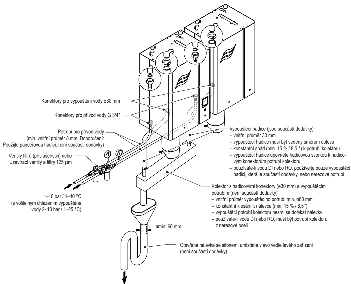
Obr. 21: Přehled vodní instalace u dvojitých jednotek Medium ("M")
