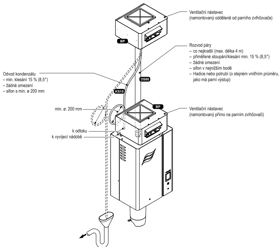
Obr. 13: Přehled instalace parního systému prostorového zvlhčování
