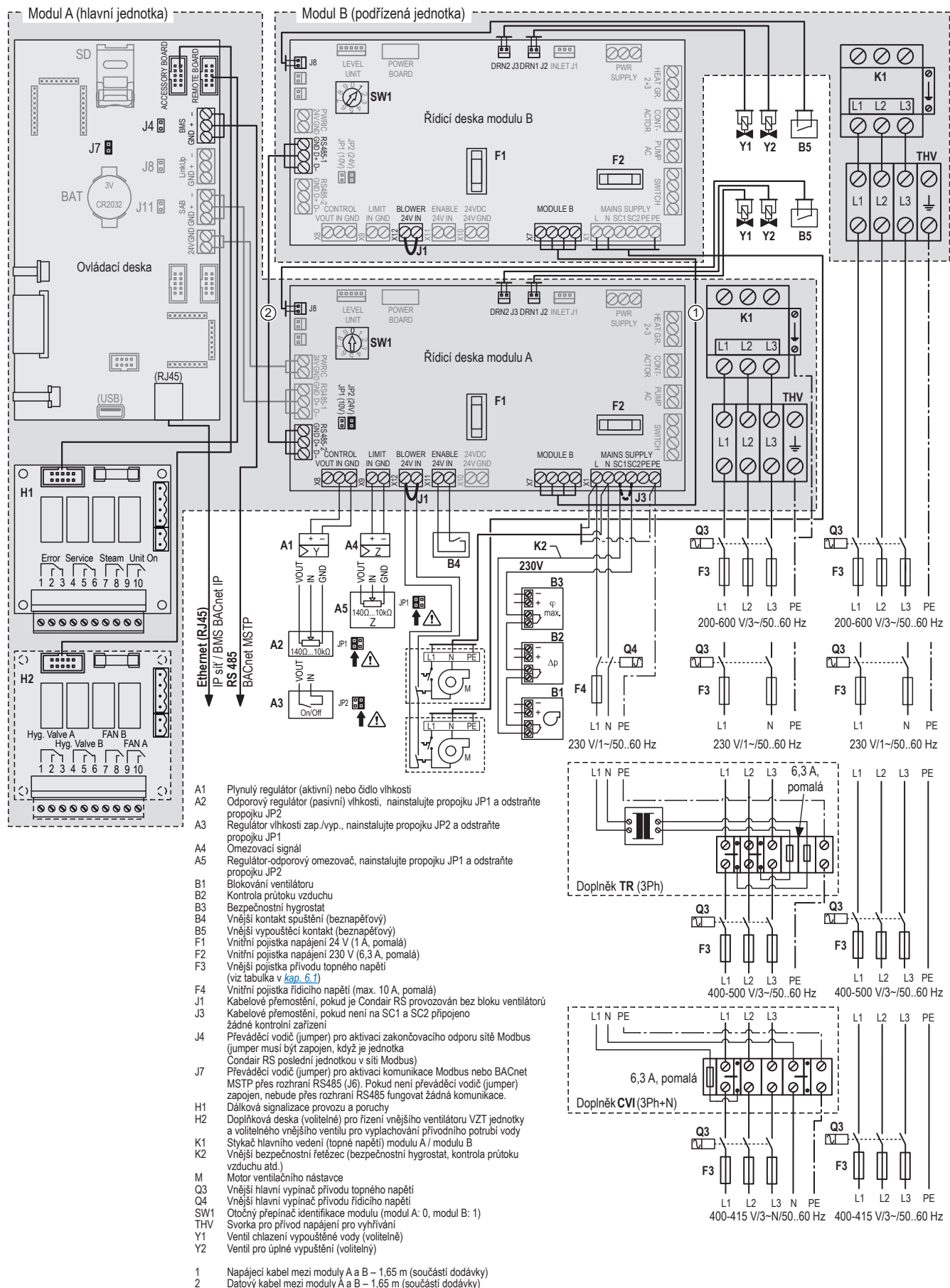
Obr. 27: Schéma elektrického zapojení dvojitých (2 x "M") jednotek Condair RS 40–80 kg/h
