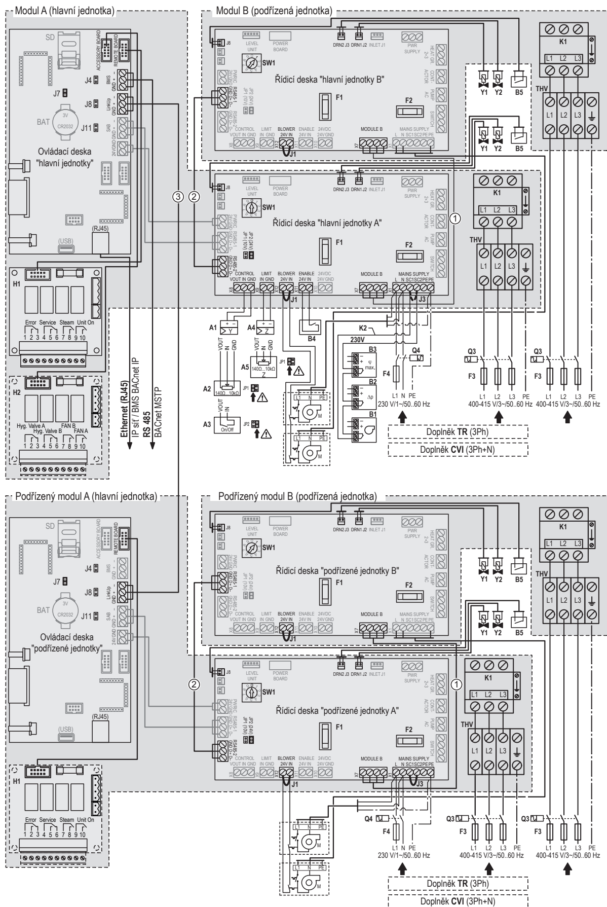
Obr. 28: Schéma elektrického zapojení systémů RS Linkup 100–160 kg/h
