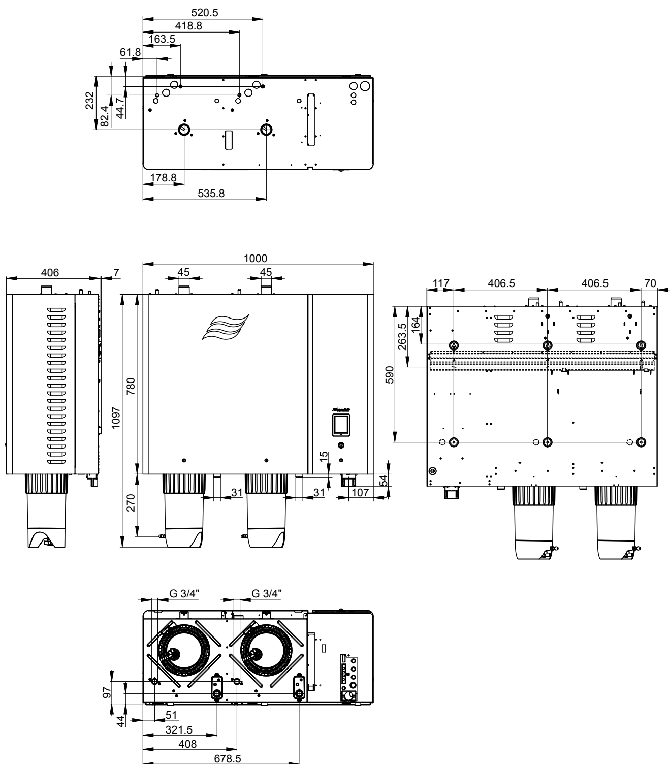
Obr. 31: Výkres rozměrů "velké" jednotky (rozměry v mm)
